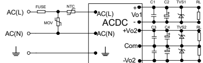
图4:AWH20-10TXXXX (三路) 系列典型应用电路
