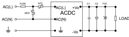
图1:AWH20-10SXXX (单路) 系列典型应用电路
