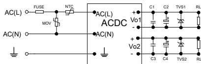
图3:AWH20-10DXXXX (双隔离双路) 系列典型应用电路
