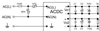
图3:AWH20-10DXXXX (双隔离双路) 系列典型应用电路
