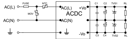
图2:AWH20-10DXX (正负双路) 系列典型应用电路
