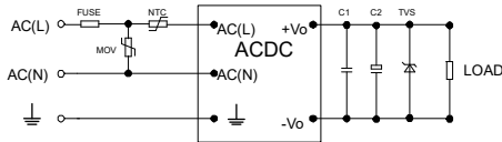
图1:AWH20-10SXXX (单路) 系列典型应用电路
