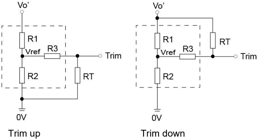
Trim 的使用电路（虚线为产品内部）
