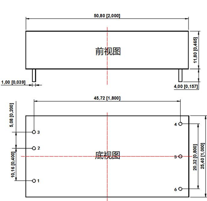
HVR60-24Sxx 系列外观尺寸图
