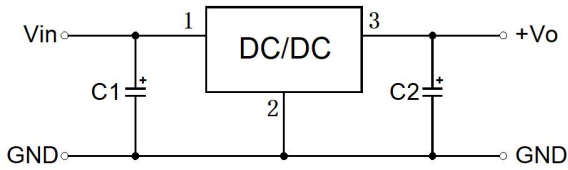
图 2-1 正输出应用电路
