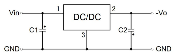
图 2-2 负输出应用电路
