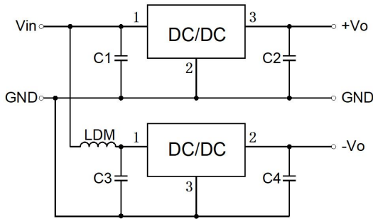
图 3 正负输出并联应用电路
