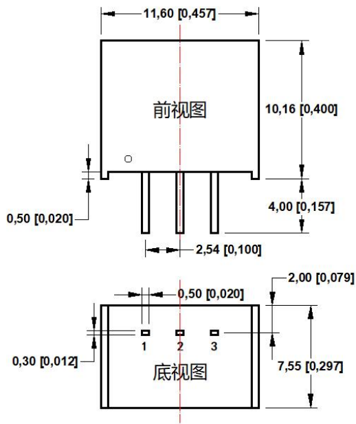
外观尺寸图
